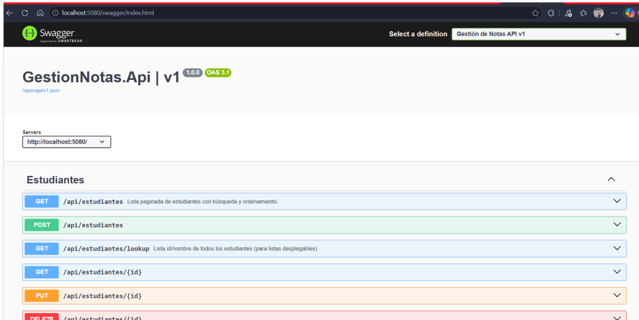
Figura 7. Swagger UI con los endpoints del API.
