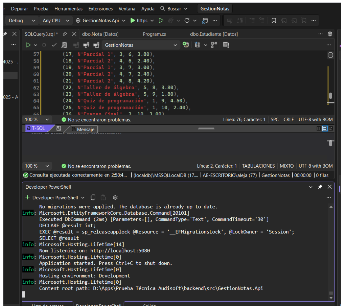
Figura 6. API en ejecución: migraciones al día y escuchando en http://localhost:5080 .
